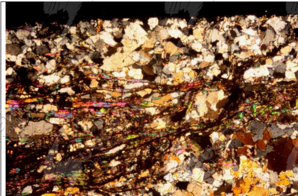
Foto 2: Foto al microscopio ottico, sezione sottile, luce trasmessa, 20 ingrandimenti, nicols incrociati
