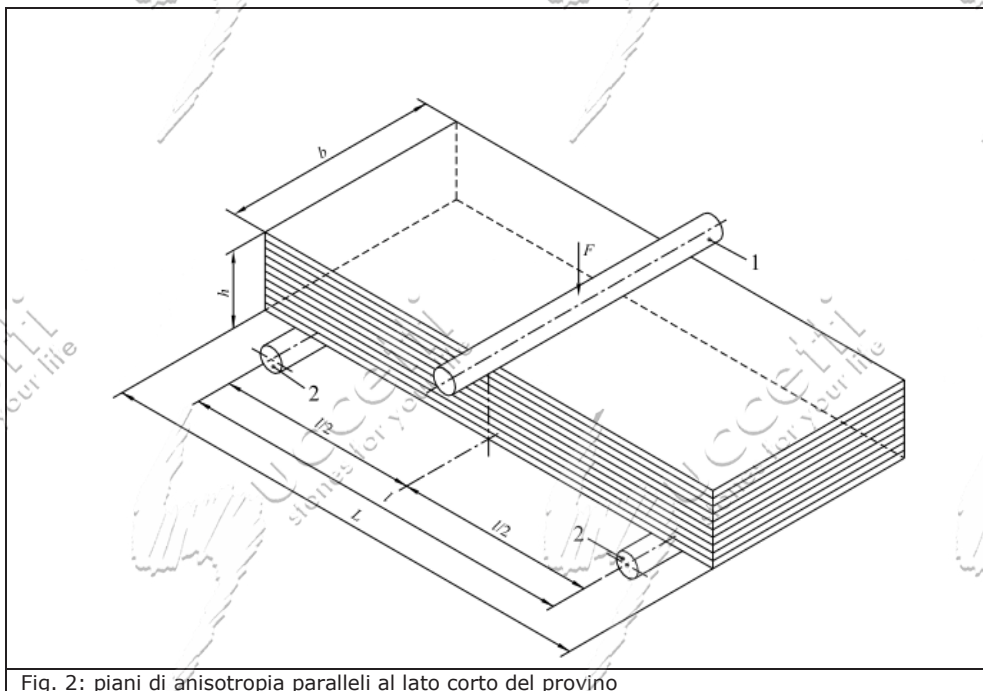
Fig. 2: piani di anisotropia paralleli al lato corto del provino
